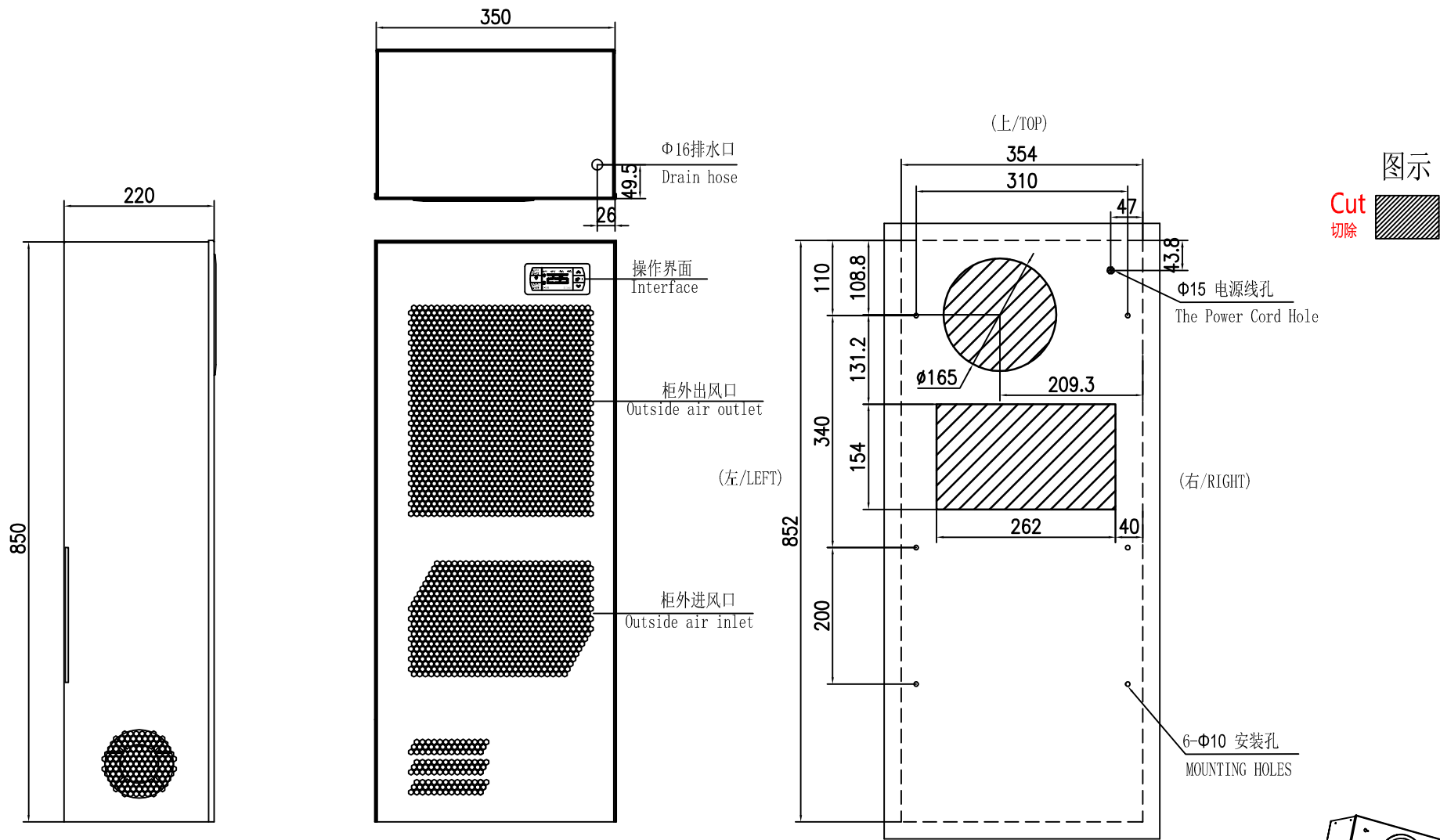
(下/BELOW) 外形尺寸和开口尺寸 Dimensions and openings dimensions
